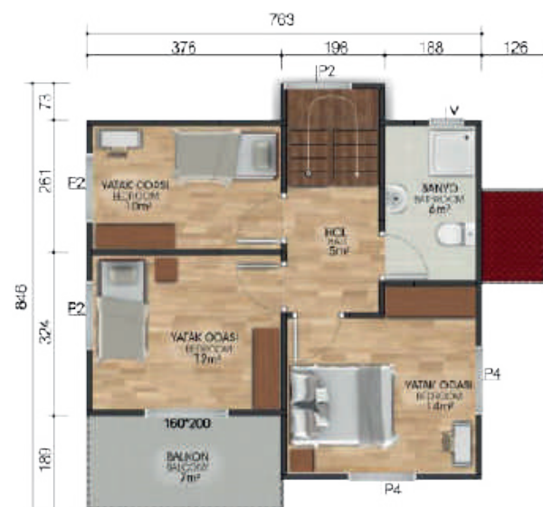
PLANTA DE DISTRIBUCIÓN SEGUNDO NIVEL
