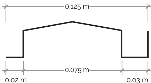
DETALLE DE PERFIL SECCIÓN TRANSVERAL
