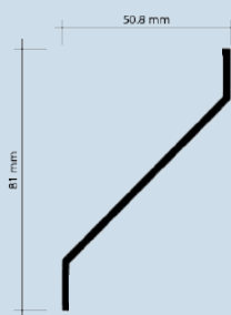
DETALLE PERFIL
